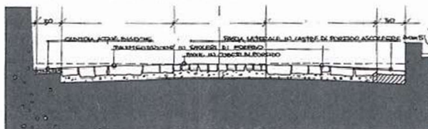
PAVIMENTAZIONE IN CUBETTI DI PORFIDO E SIOXEDI
