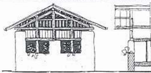
SESTIA ELEMENTI STRUTTURALI IN LEGNO TRADIZIONALI
