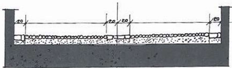
PAVIMENTAZIONE IN CIOTOLIATO
