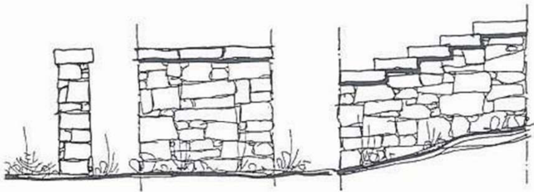
MURETTI DI RECINZIONE IN PIETRA LOMEA FACCIA A VISTA CON CORSETTINA IN LASTRE
