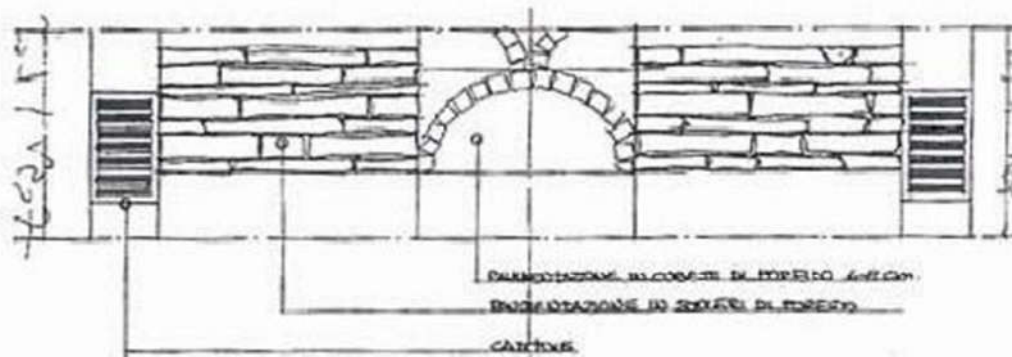
PAVIMENTAZIONE IN COSETE DI PORFIDO POSATE AD ARCHI CONTRASTANTI
