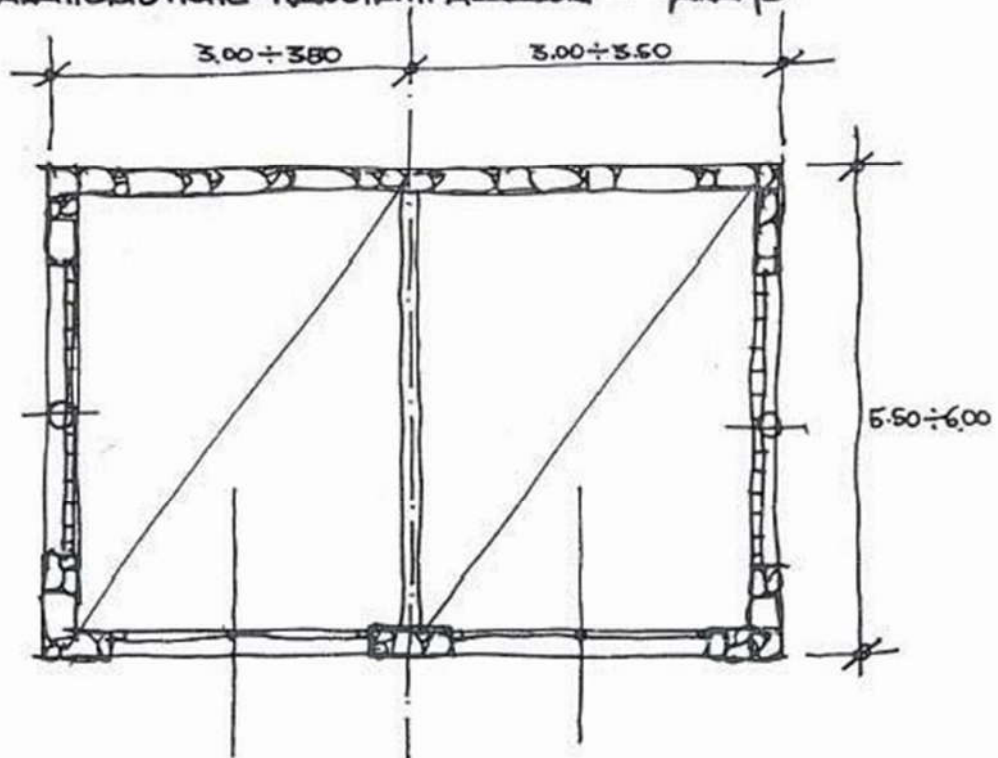
CARATTERISTICHE MANUFATTI ACCESSORI - GARAGE -
