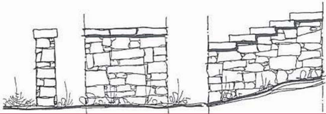
MURETTI DI RECINZIONE IN PIETRA LOCALE, FACCIA A VISTA CON COPERTINA IN LASTRE
