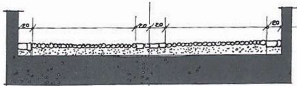
PAVIMENTAZIONE IN CIOTOLI
