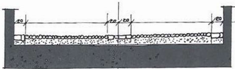
PAVIMENTAZIONE IN CIOTOLATO
