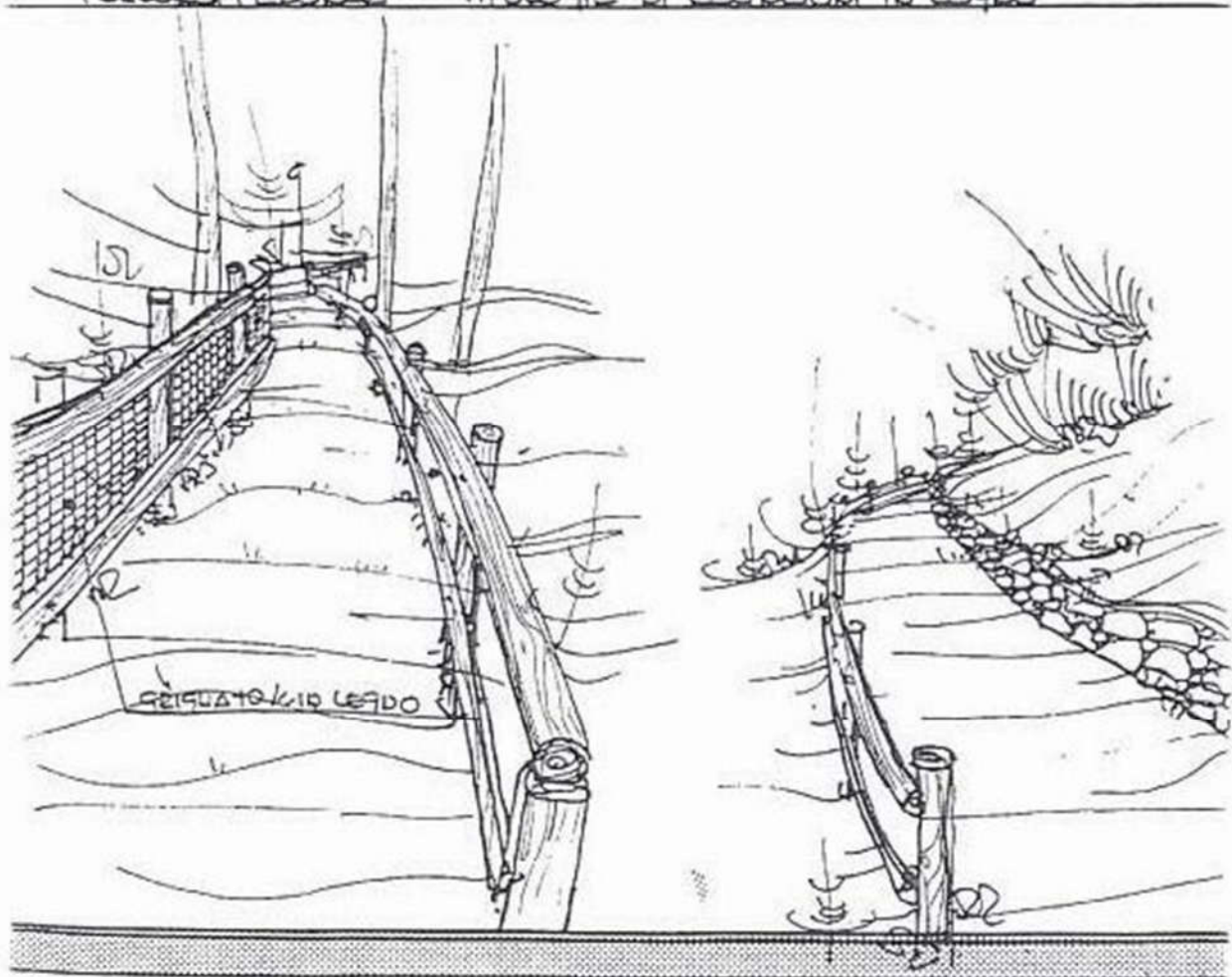
PERCORSI PEDONALI - TIPOLOGIE DI RECINZIONI IN LEGNO
